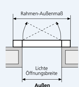
Einbau hinter der Laibung
