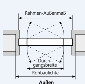
Einbau zwischen der Laibung*
