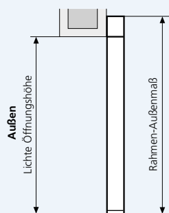
Einbau hinter der Laibung*
